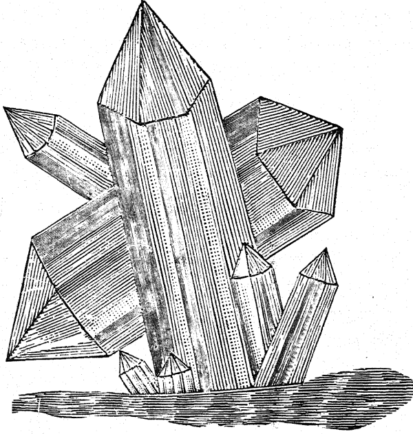
चित्र १५३—स्फटिक मणि ( काट्टंज )
